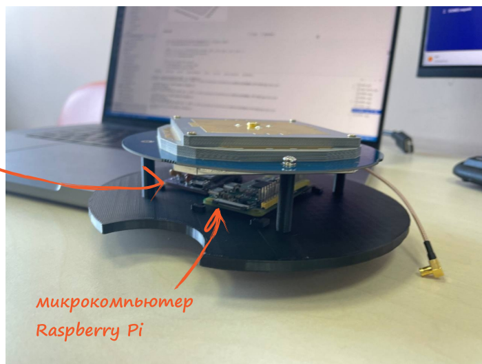
ГНСС-чип U-Blox
